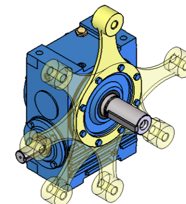
Braço de torção
