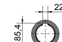
Detalhe C Eixo de saída vazado
